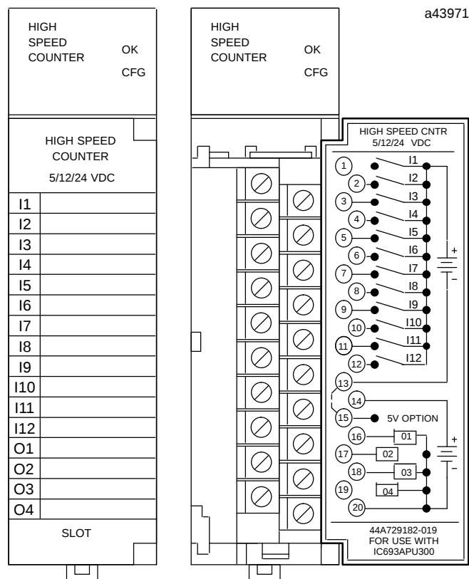
Abbildung 1-1 Schnelles Zählermodul der Serie 90-30
