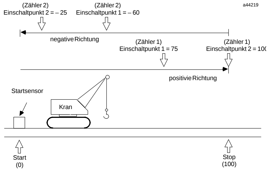
Abbildung A-1 Beispiel von richtungsabhängiger Erfassung
