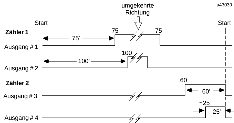
Abbildung A-2 Ausgangs-Zeitverhalten
