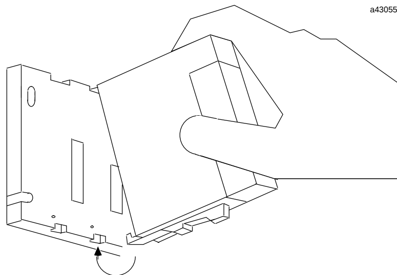
Abbildung 2-1 Einbau eines Serie 90-30 Moduls
