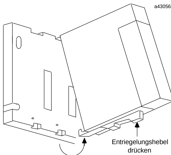
Abbildung 2-2 Ausbau eines Serie 90-30 Moduls
