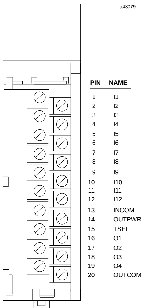
Abbildung 2-4 Anschlußbelegung des Klemmenteils
