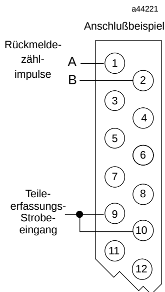
Abbildung A-6 Beschaltungsbeispiel
