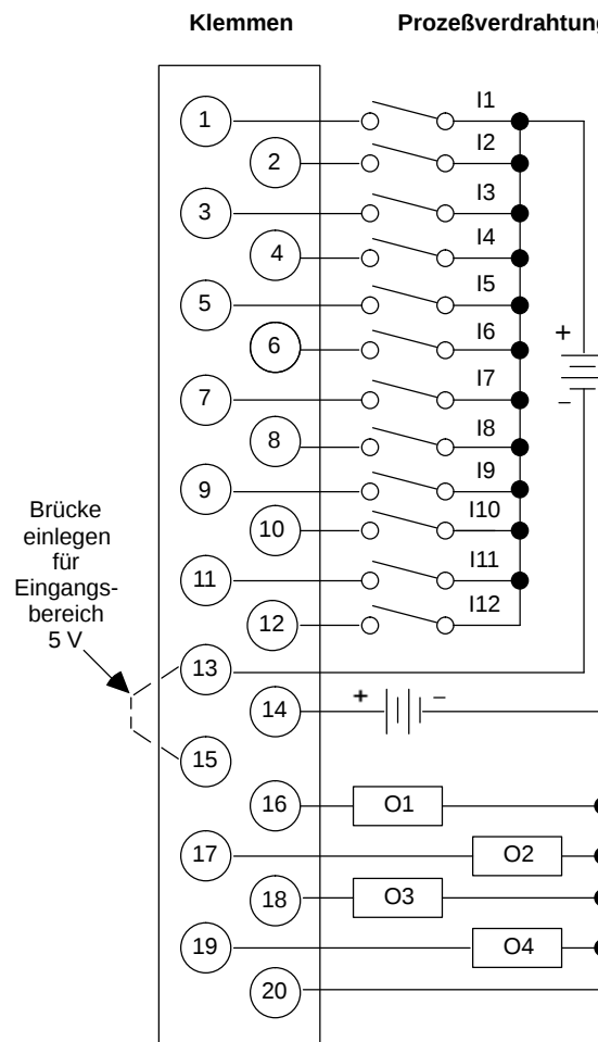
Abbildung 2-5 Anschlußbeschriftung des schnellen Zählermoduls
