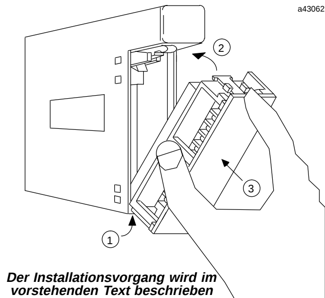
Abbildung 2-3 Einbau des Klemmenteils
