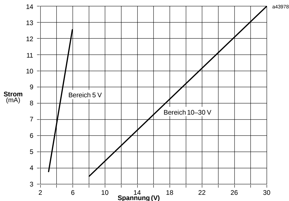
Abbildung 1-2 Strom-/Spannungscharakteristik der Eingänge
