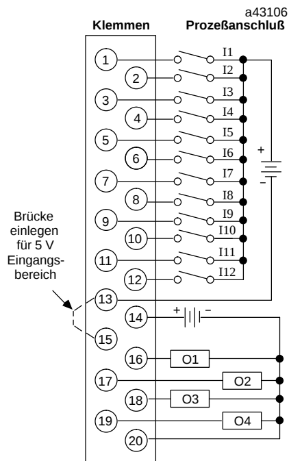
Abbildung B-1 Anschlußbeschriftung des schnellen Zählermoduls
