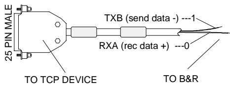
HMI-CAB-C98
