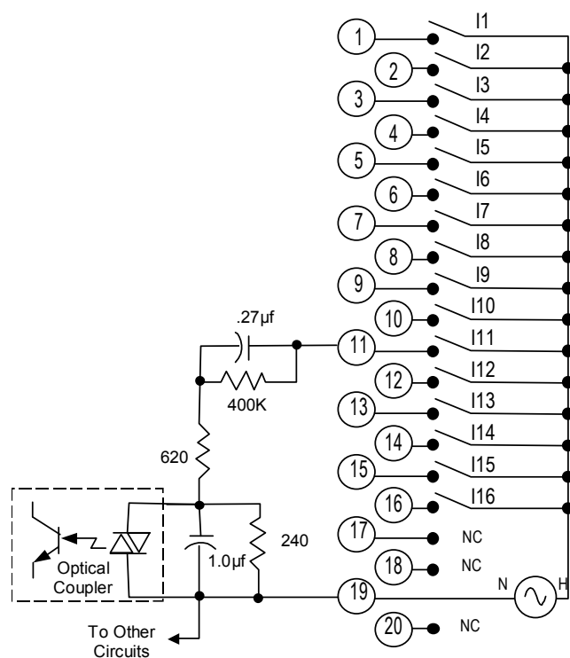
Module Circuits
